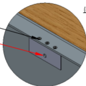
DETAIL A SCALE 1 : 5 Aluminium slotvoorbereiding 100 x 40 x 20 mm
